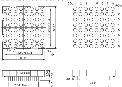
BL-M23D881RGB (BL-M23C881RGB C.C.)
